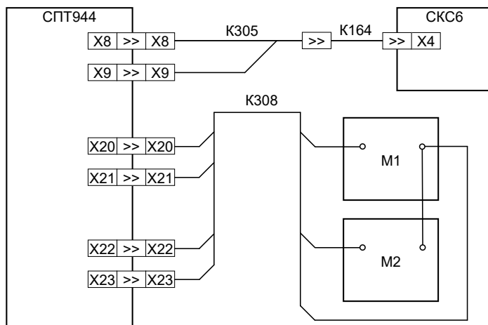
Рисунок 11.2 – Схема проверки
