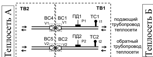
Рисунок В.4 – Схема с двумя реверсивными расходомерами для учета на границе смежных тепловых сетей и на переключках
